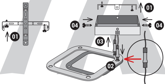
FIGURA 1 - Montare piciorușe și fixare sistem de prindere de lustră
